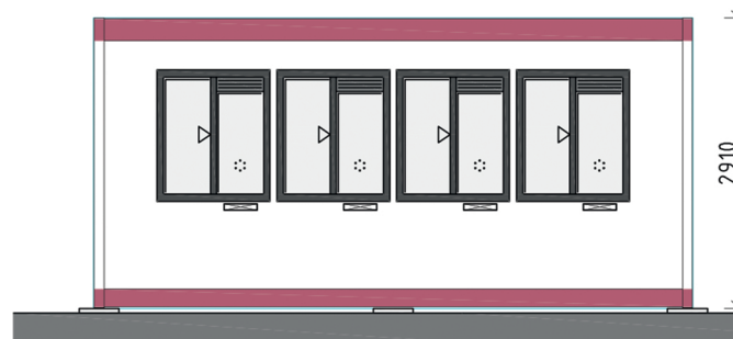
Gevelaanzicht loketzijde
