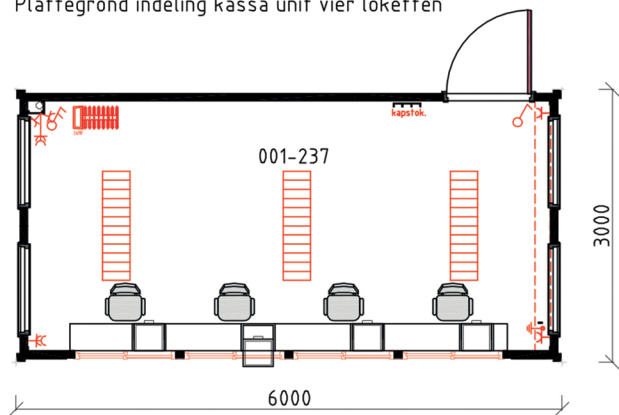
Plattegrond indeling kassa unit vier loketten
